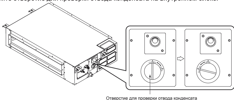
Отверстие для проверки отвода конденсата
